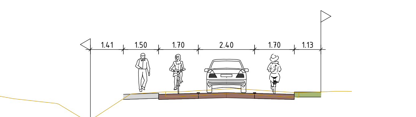
Normaalprofiel binnen bebouwde kom
