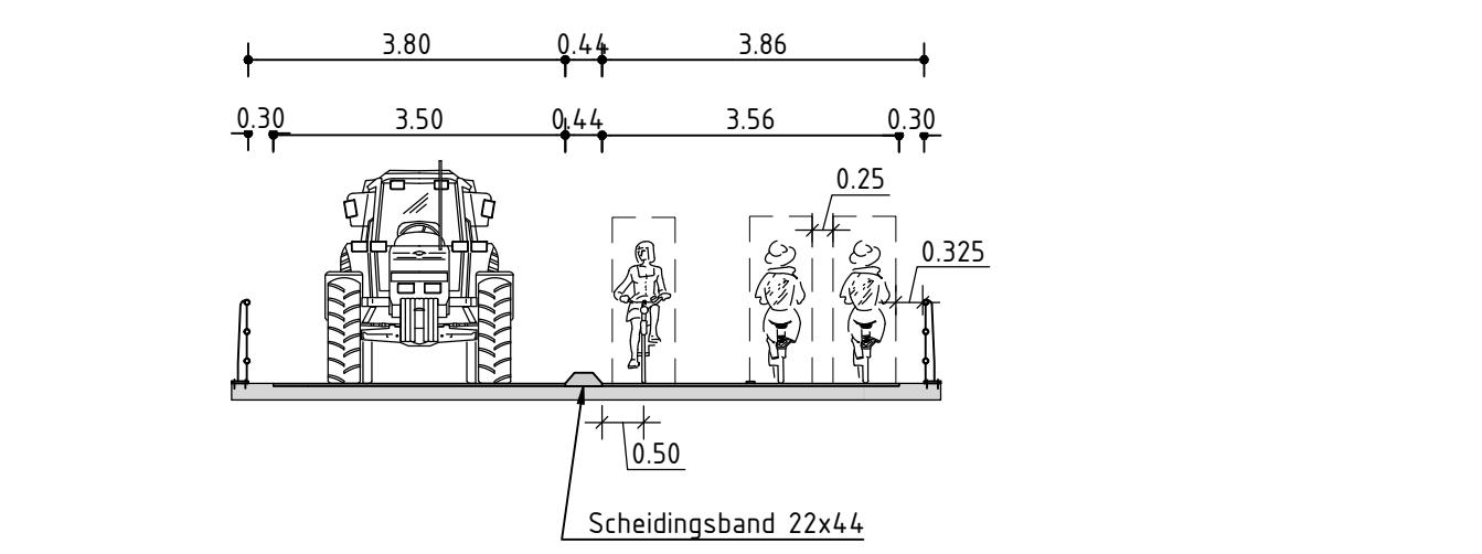
Profiel om-en-om-regeling viaduct A15
