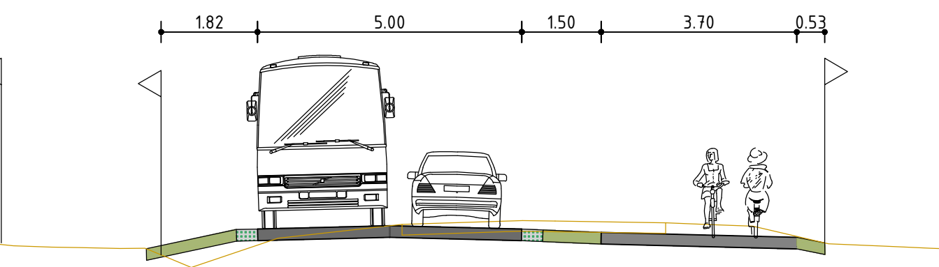
Normaalprofiel buiten bebouwde kom
